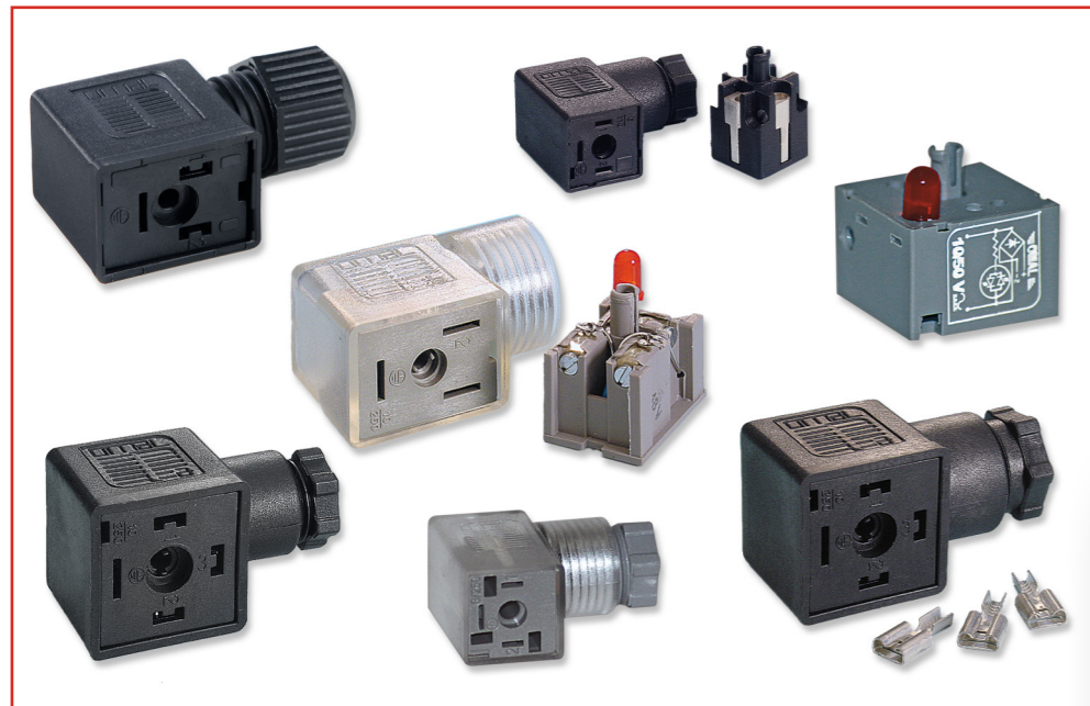
Connettori a cablare Field-wireable connectors Selbstanschließbare Ventilstecker EN 175301 - 803
